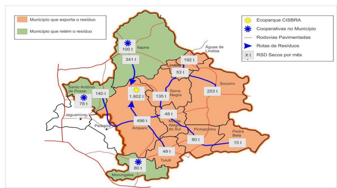
Figura 4 - Fluxo mensal de RSD Secos - CISBRA
