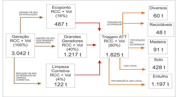
Figura 28 - Fluxograma mensal dos RCC - Município de Amparo
