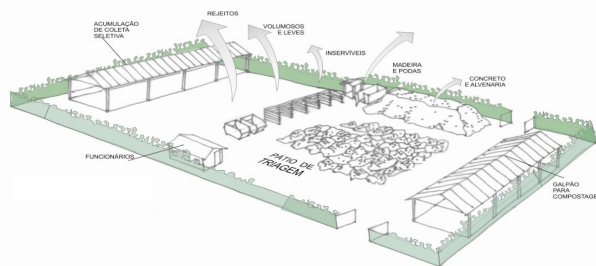
Figura 14 - Desenho ilustrativo do Ecoponto/ATT – área em torno de 3.600 m 2
