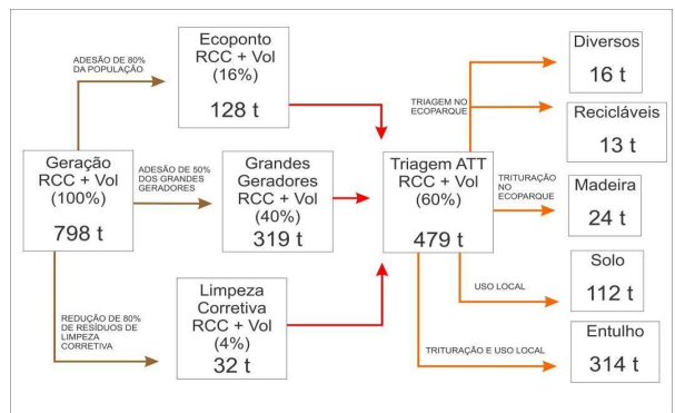
Figura 26 - Fluxograma mensal dos RCC - Município de Águas de Lindoia
