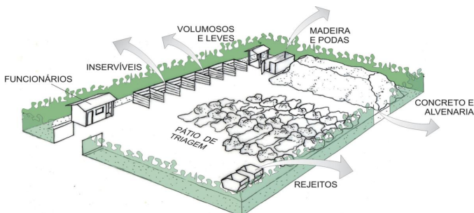
Figura 13 - Desenho ilustrativo da Área de Triagem e Transbordo – ATT – área em torno de 2.000m 2
