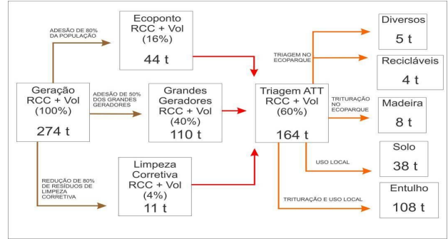
Figura 48 - Fluxograma mensal dos RCC - Município de Tuiuti
