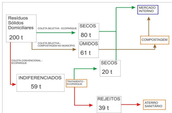
Figura 39 - Fluxograma mensal dos RSD - Município de Pinhalzinho
